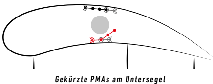
Gekürzte PMA's am Untersegel
