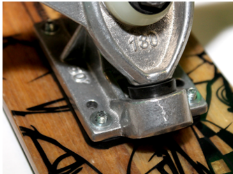
4. Unterlegscheiben aufsetzen und Muttern festziehen
